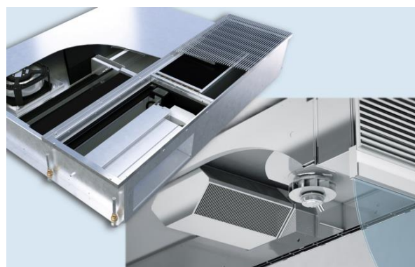
Weitere Neuerungen im Bereich dezentrale Klimatisierung: die Fassadenlüftungsgeräte FVP PulseVentilation (oben) und FVS Eco2School (unten).
