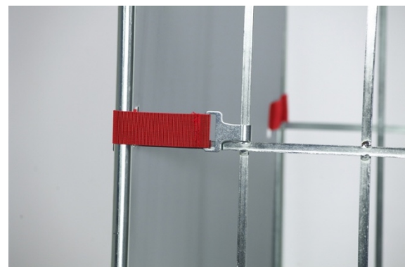
Die Haken werden an den Vertikalstreben des Rollcontainers befestigt.
